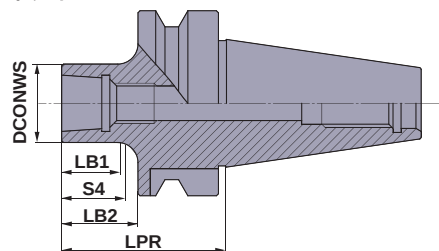
ストレートタイプ
